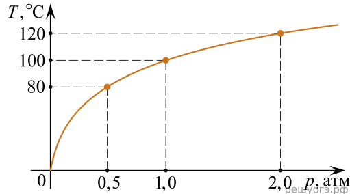
Зависимость температуры кипения воды от давления
