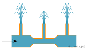
Протекание жидкости через трубу с сужением
