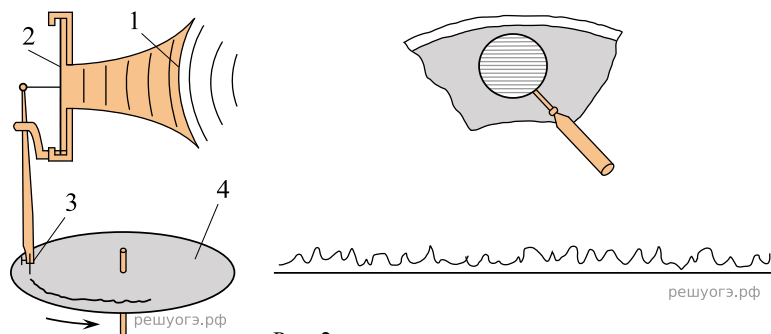
Рис. 2 Профиль звуковой дорожки на фонографе при большем увеличении
