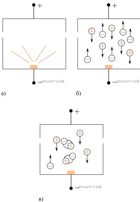
Принцип действия ионизационного извещателя
